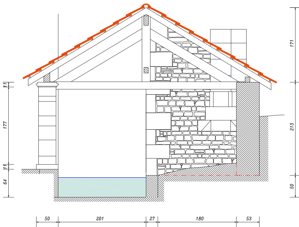
Vue en élévation suivant coupe AA'
