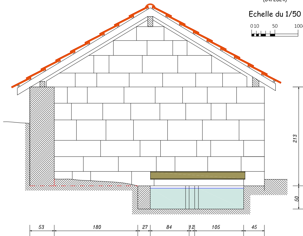
Vue en élévation suivant coupe BB'
