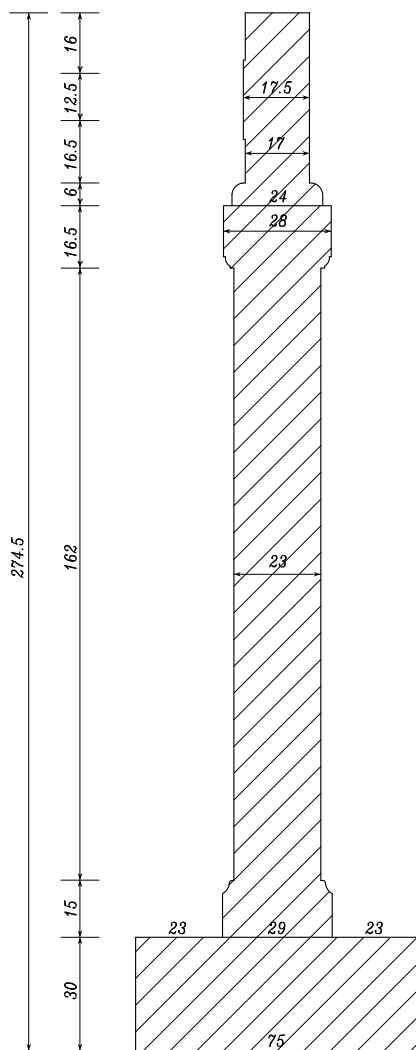
Coupe longitudinale
