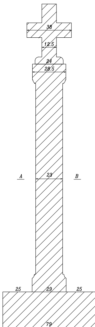
Coupe transversale
