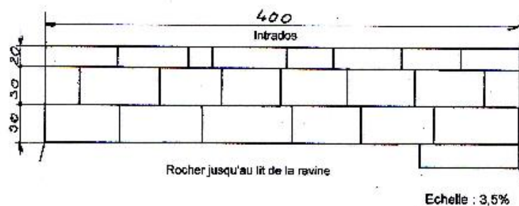
Assises ouest
