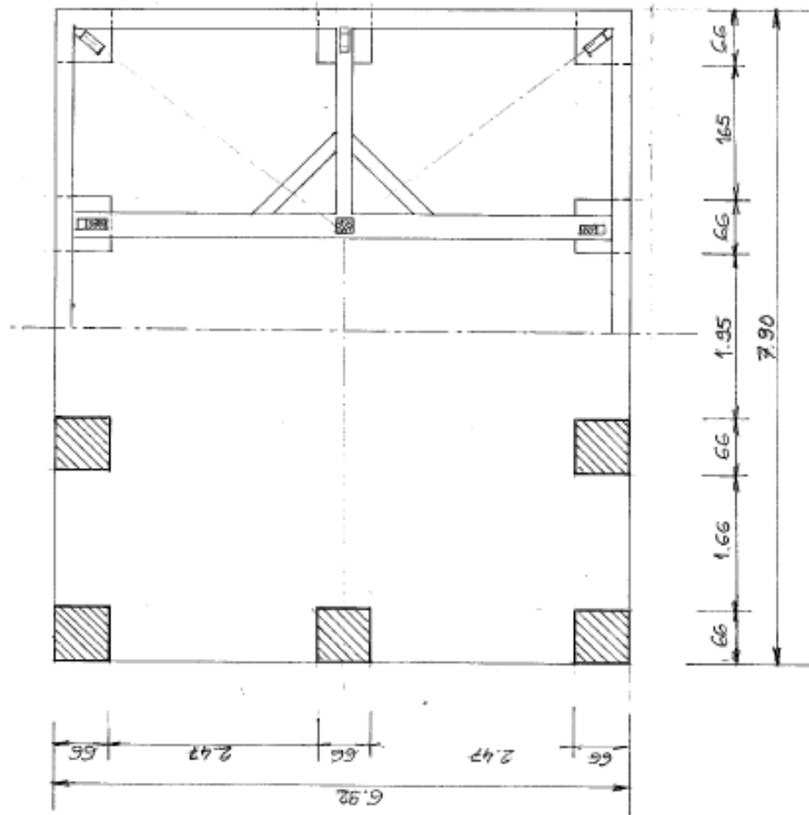
Vue en plan, coupe sur piliers et coupe au dessus des poutres
