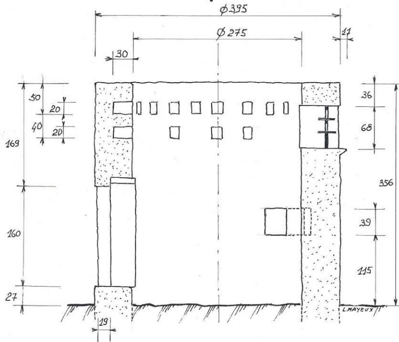
Lucarne d'envol Ech 1/20
