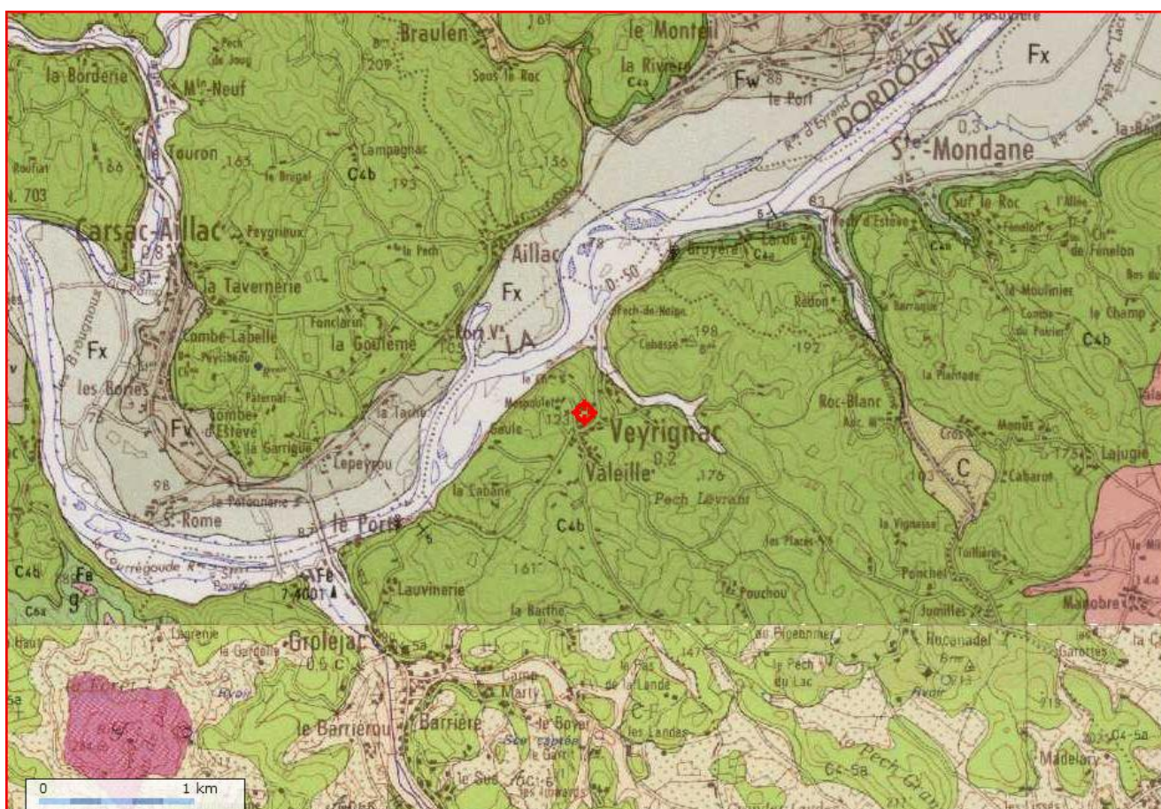
Légende : les zones vertes notées C2 correspondent au crétacé supérieur
