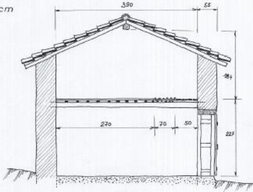
Coupe schématique des clés
